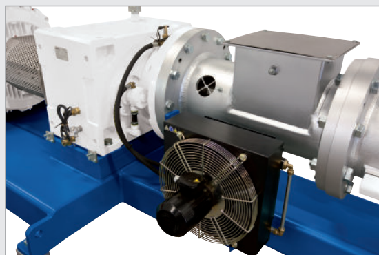
Привод с комбинированным узлом редуктора и подшипника
