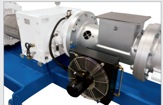
Aandrijving met gecombineerde lagering en reductiekast
