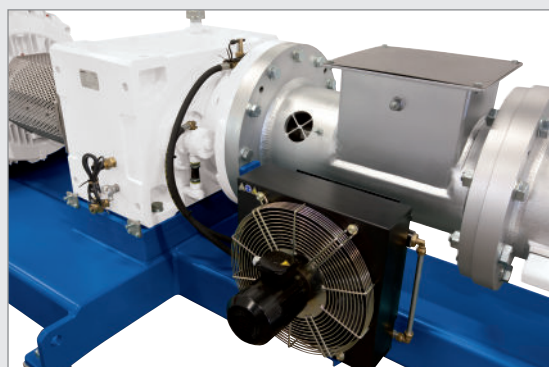
Entraînement avec ensemble combiné boîte de vitesses-palier
